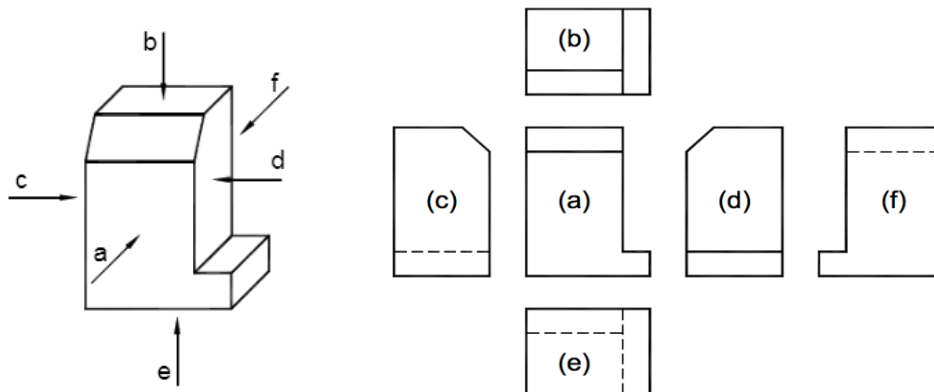
Figura 9. Vistas – Uso de la línea punteada 12
