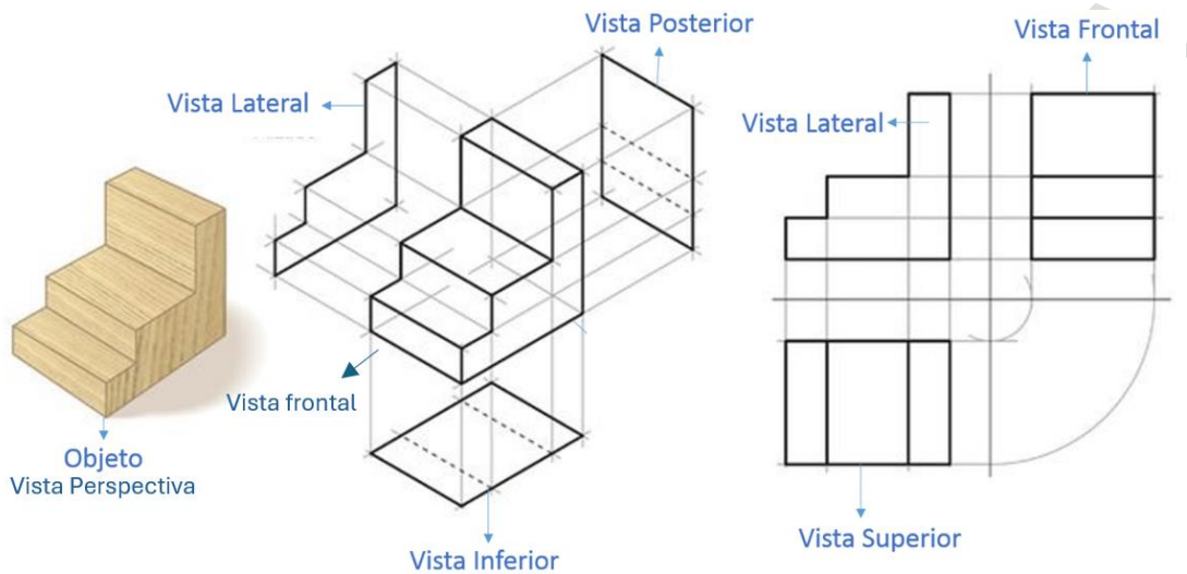
Figura 6. Designación de las vistas 9
